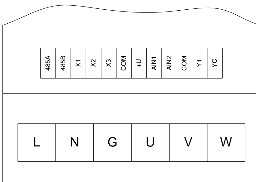
Рисунок 5 – Расположение клемм ПЧ
