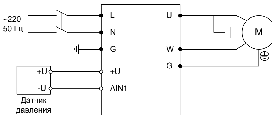
Рисунок 4 – Схема подключения ПЧ
