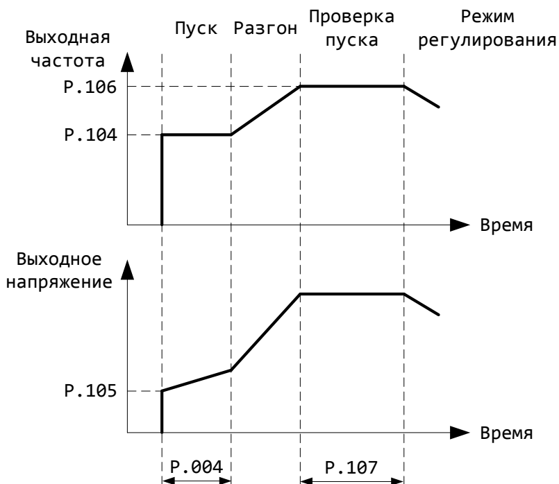
Рисунок 9 – Диаграмма работы ПЧ в режиме пуска
