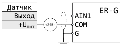
Рисунок 8 – Типовые схемы подключения аналоговых входов AIN
